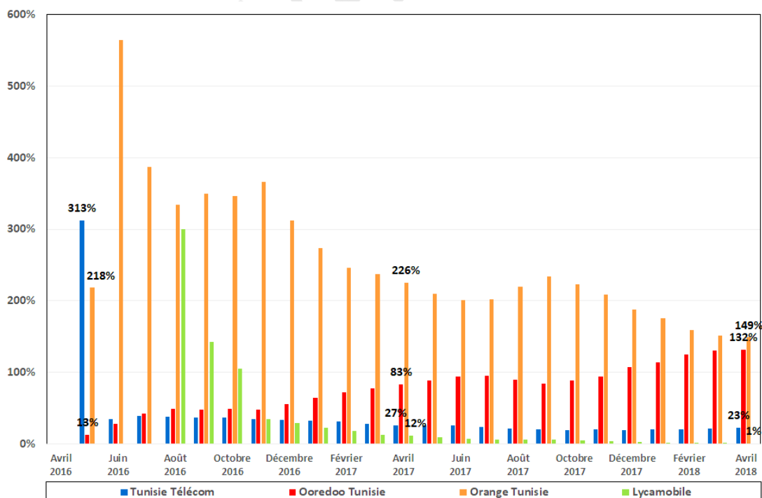
Fig30 : Evolution mensuelle du ratio Entrant/Sortant par opérateur.
